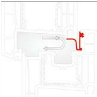
Hanóaszélnyomás, a REHAU AirComfort a Bernoulli-elvszerint automatikusan bezárul
